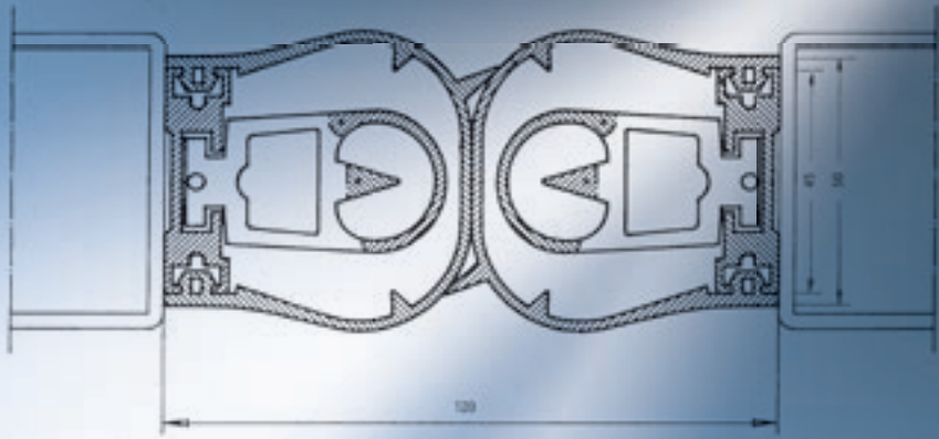
Gummihüllprofil in der Anwendung – Hauptschließkante mit Sicherheitsleiste in eingebautem Zustand. Benötigte Materialien: siehe rechte Seite
