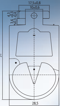
Contact-Duo-Profil 016.10
