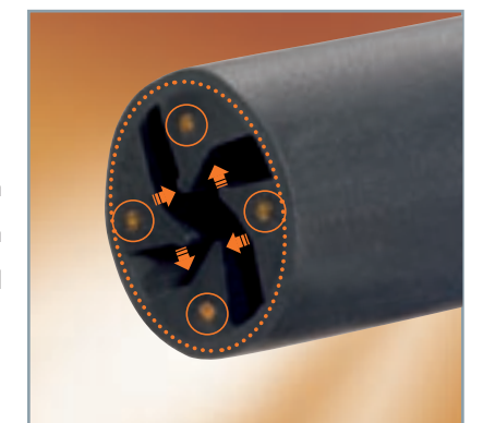
Gelbau Quadro-Profil
