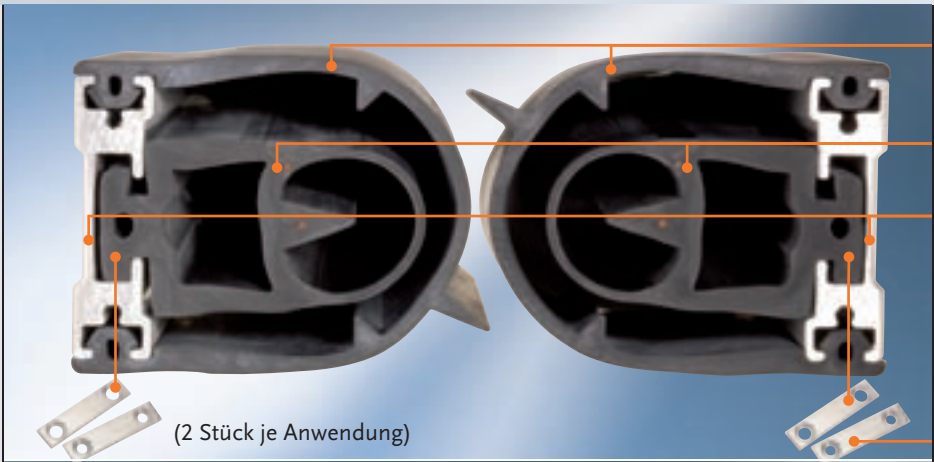
Gummihüllprofil in der Anwendung – Hauptschließkante mit Sicherheitsleiste in eingebautem Zustand. Benötigte Materialien: siehe rechte Seite
